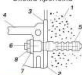
Схема крепежа
